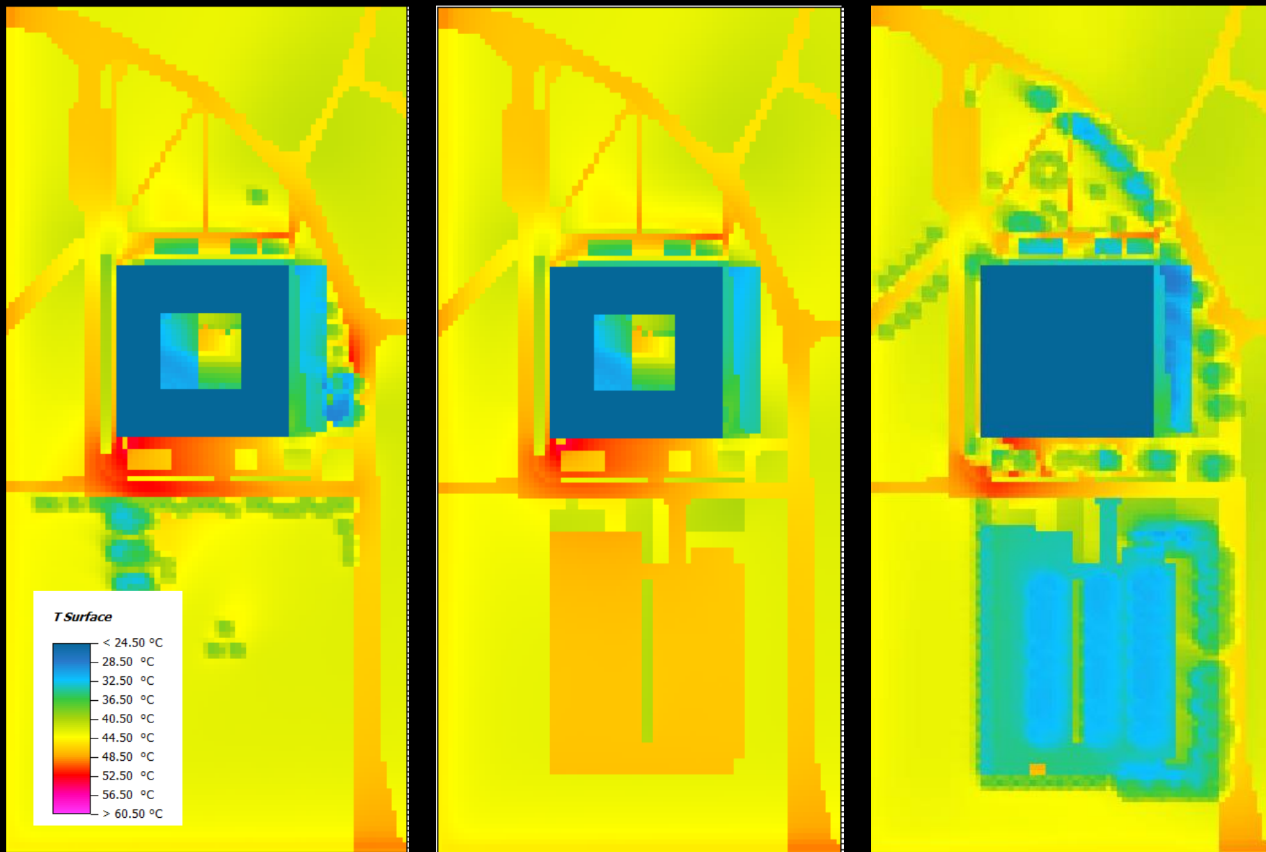
Povrchová teplota 14 hod.
