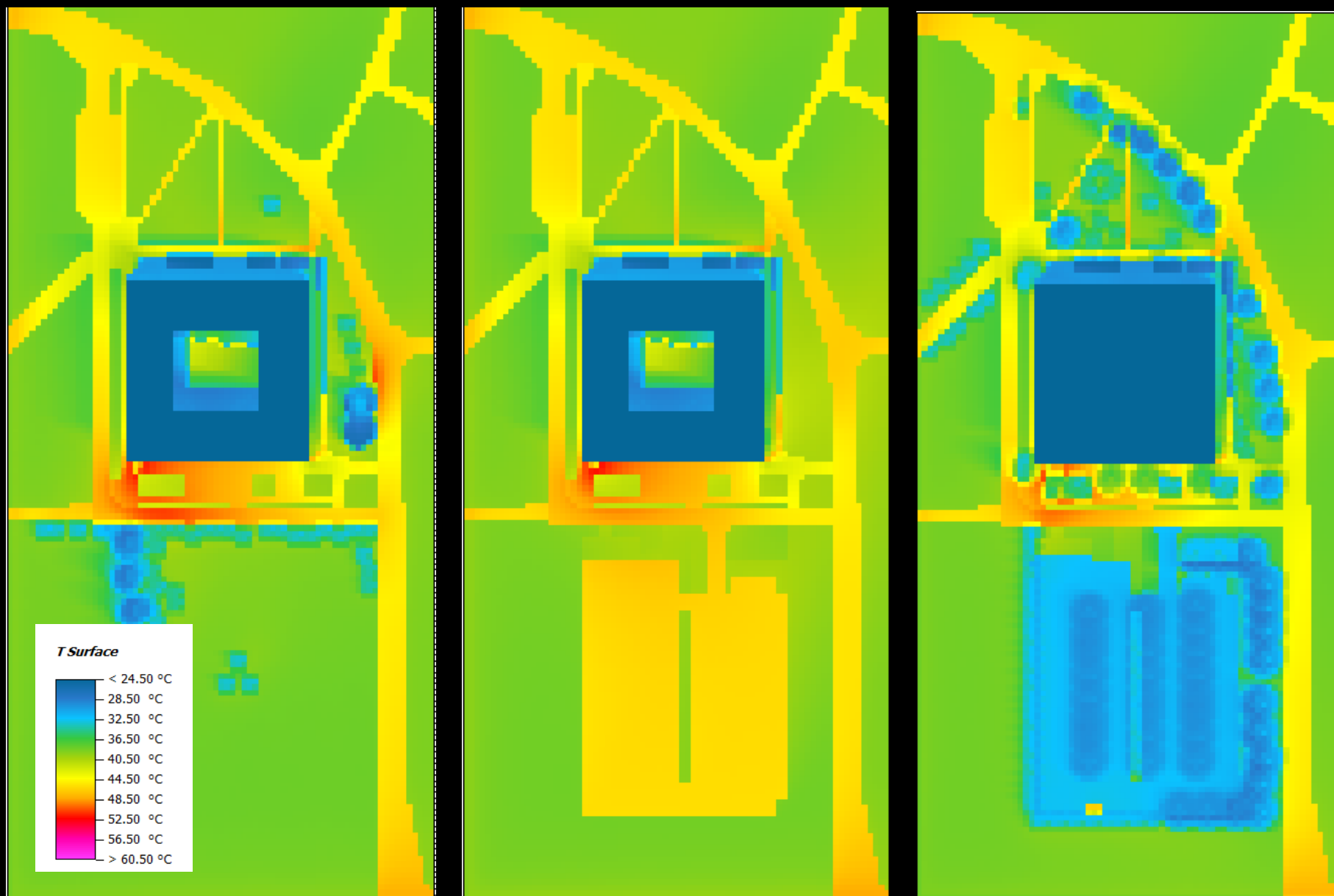
Povrchová teplota 12 hod.
