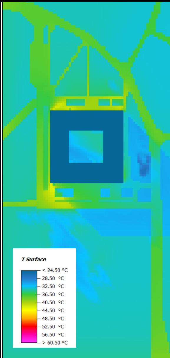
Povrchová teplota 18 hod.
